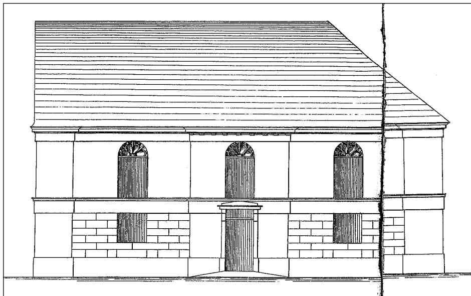
Widok na boczną elewację pierwotnego projektu kościoła ewangelickiego w Dobrzycy autorstwa krotoszyńskiego inspektora budowlanego Tollkemitha z 1805 r. Archiwum Państwowe w Poznaniu, Konsystorz Ewangelicki, sygn. 3939
