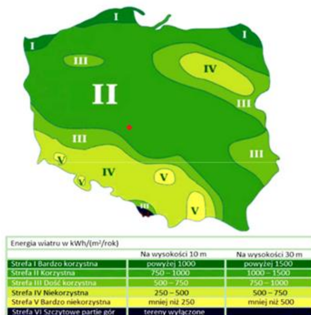
Ryc. 12. Energia wiatru w Polsce w kWh/(m²/rok) na wysokości 10 i 30 metrów
